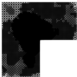
Fig. 4.2a: Reentrant corner
